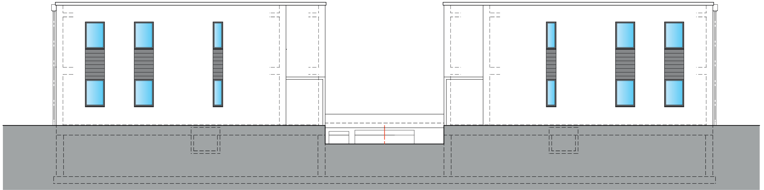
Ansicht Ostseite
